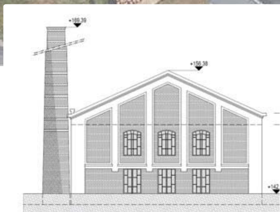
PROSPETTO DI PROGETTO NORD
