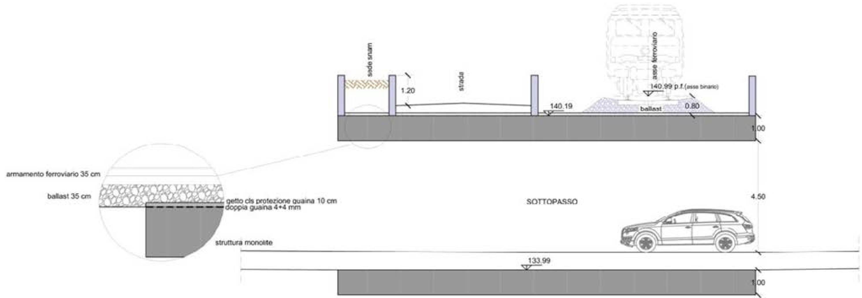
SEZIONE LONGITUDINALE TIPO MONOLITE
