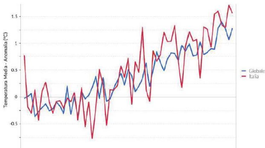
Figura 205: Serie delle anomalie di temperatura media globale sulla terraferma e in Italia, rispetto ai valori climatologici normali 1961-1990.
