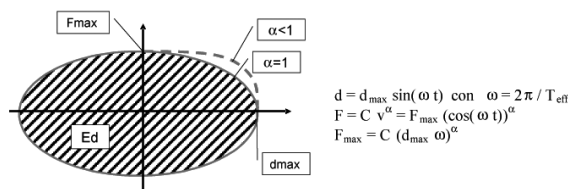
Fig. 11.9.2 – Dispositivi a comportamento viscoso
