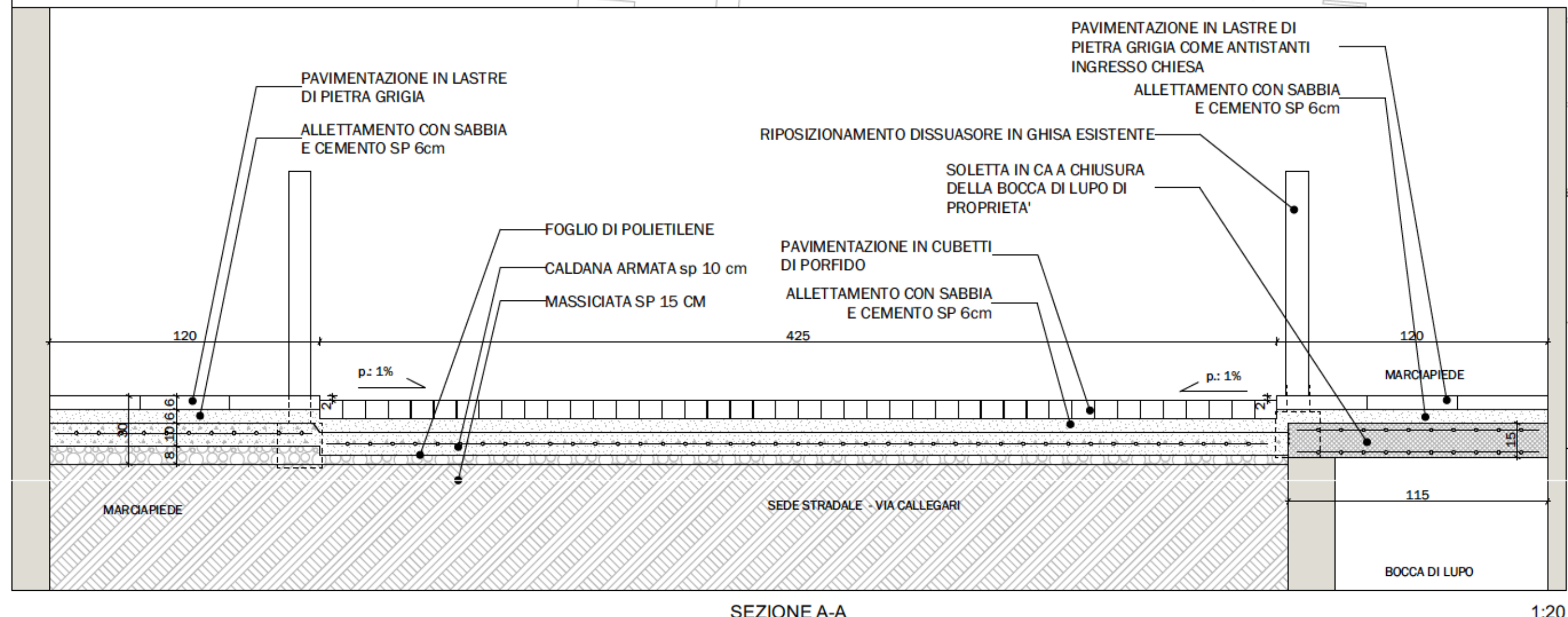
SEZIONE A-A
