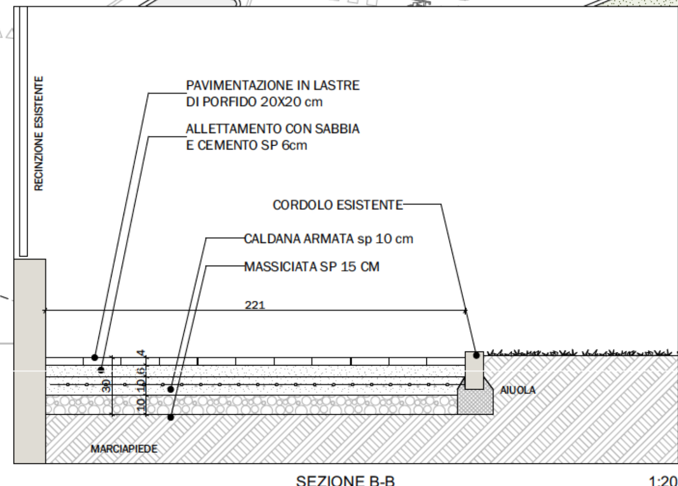
SEZIONE B-B
