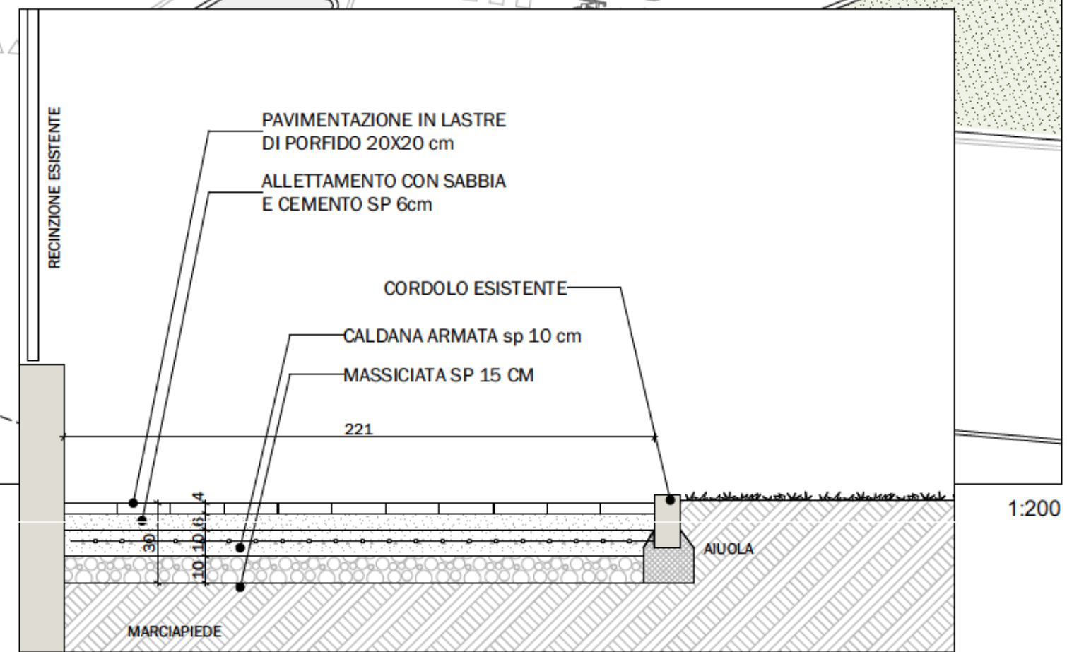
SEZIONE B-B
