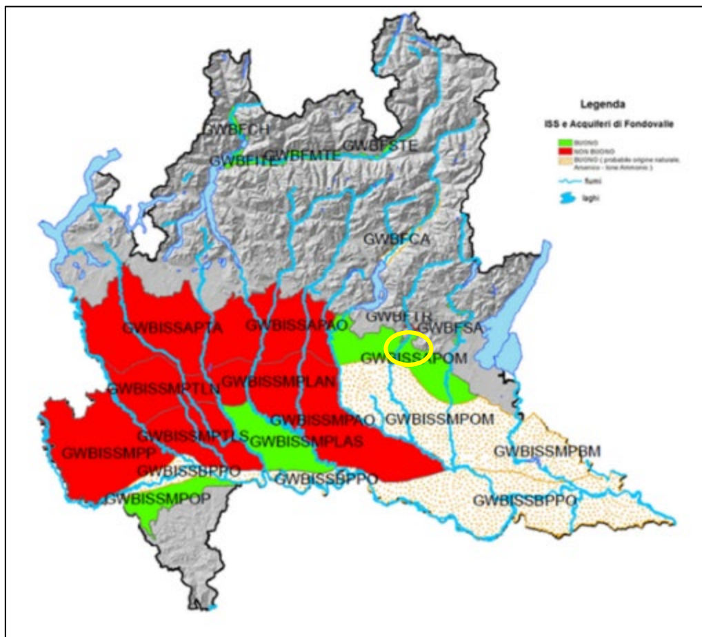
Corpi idrici sotterranei – Idrostruttura Sotterranea Superficiale e Fondovalle - Stato Chimico 2014-2019
