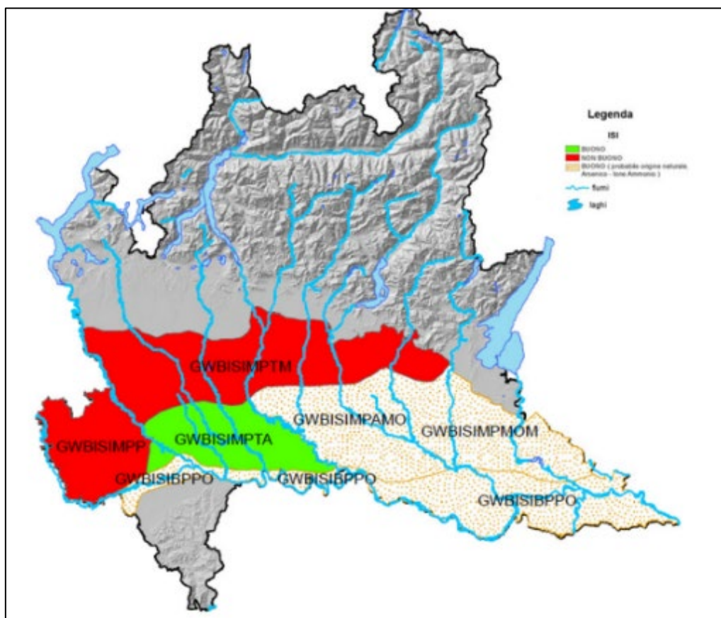
Corpi idrici sotterranei – Idrostruttura Sotterranea Intermedia - Stato Chimico 2014-2019
