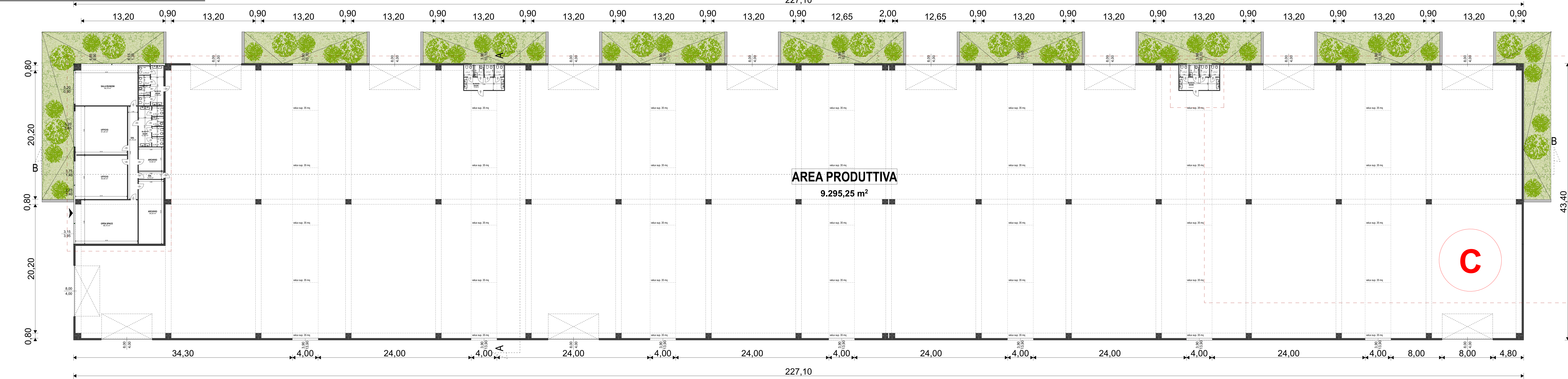
PIANTA PIANO TERRA 1:200
