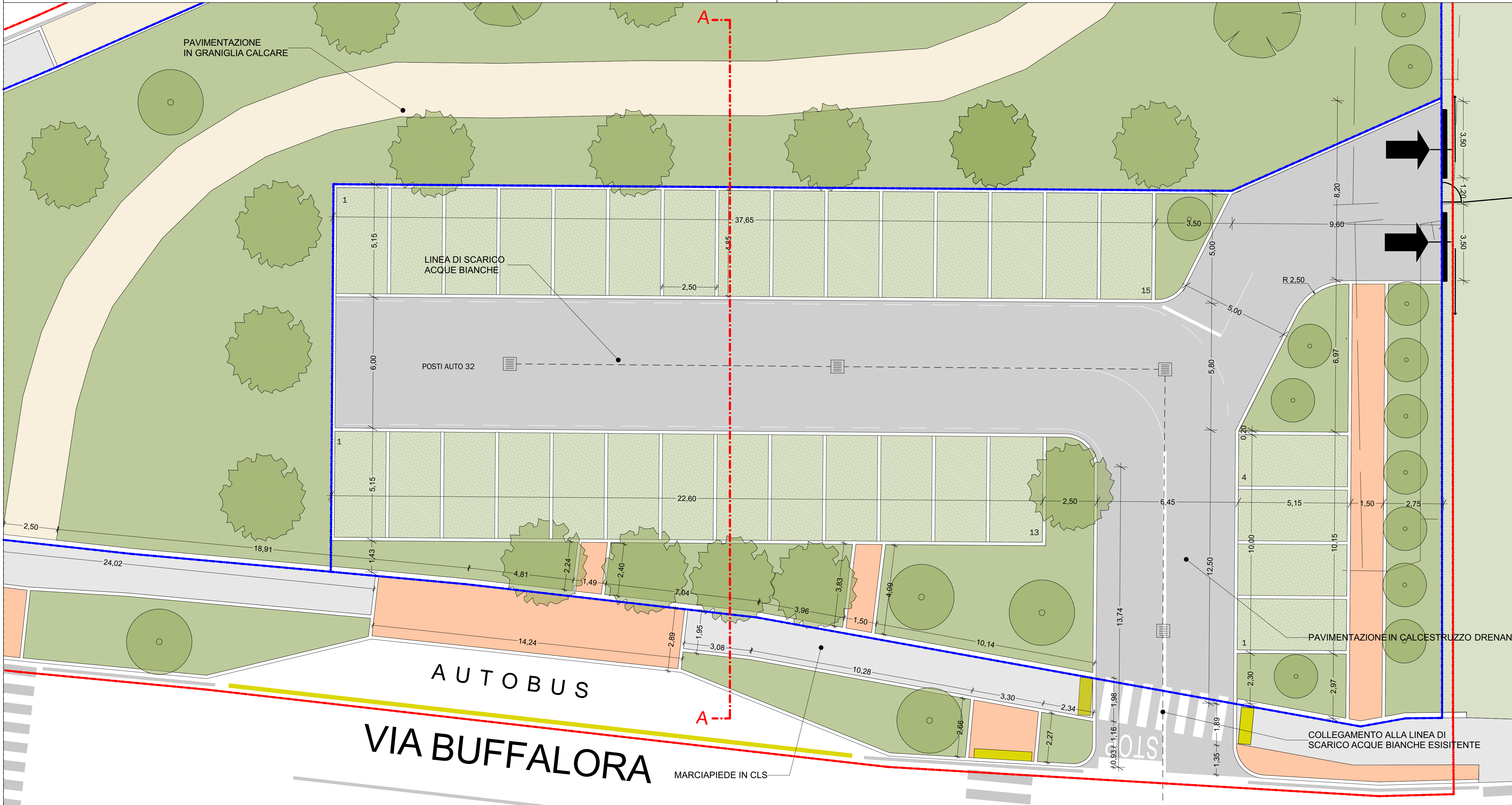
PLANIMETRIA DI DETTAGLIO PARCHEGGIO
