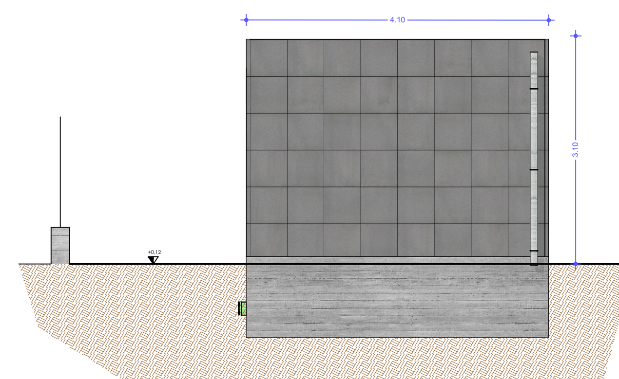
prospetto lato - vista dal marciapiede
