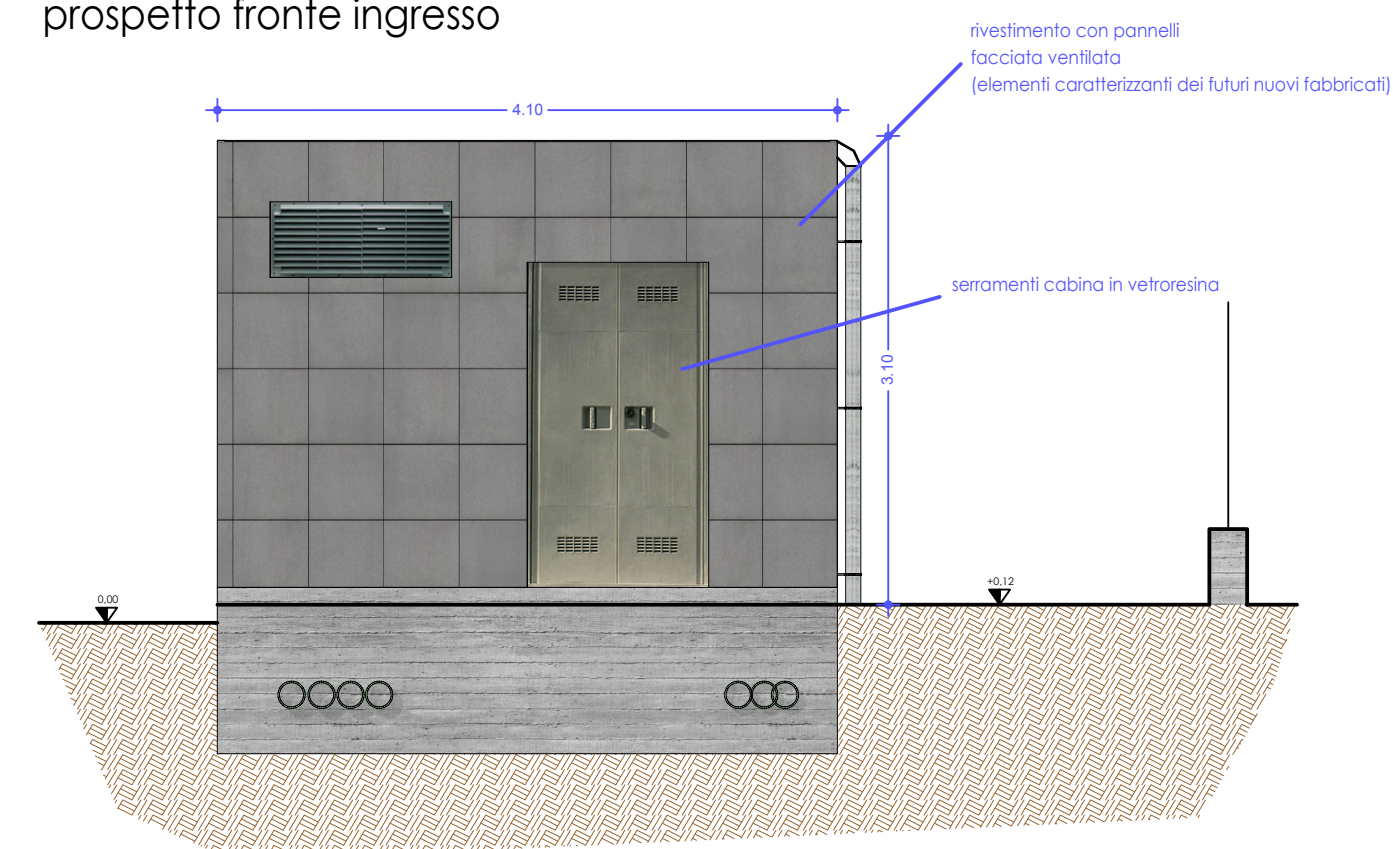
prospetto fronte ingresso
