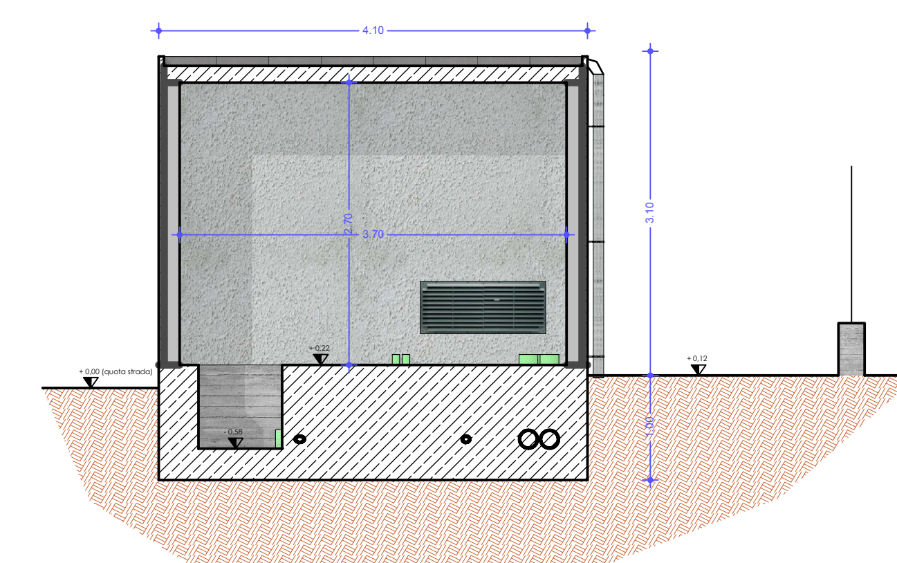
sezione x-x
