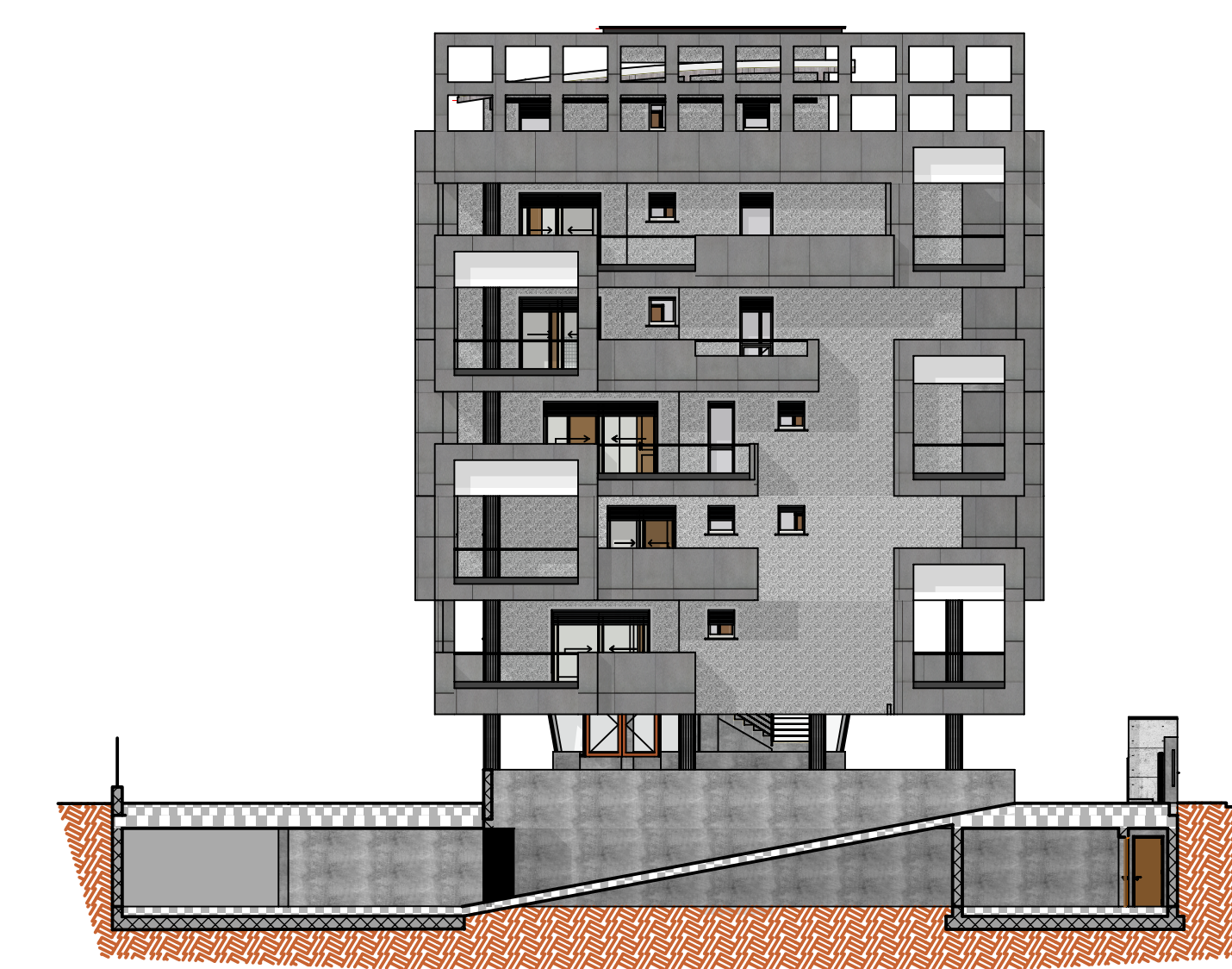
PROSPETTO SUD-EST (VISTA LATO)
