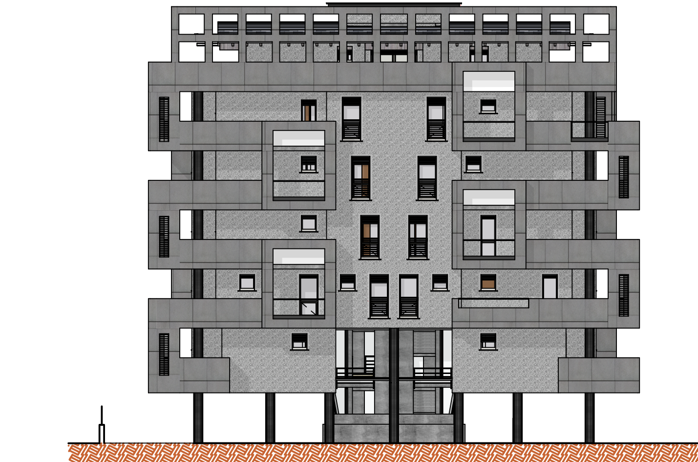
PROSPETTO SUD-OVEST [VISTA RETRO]
