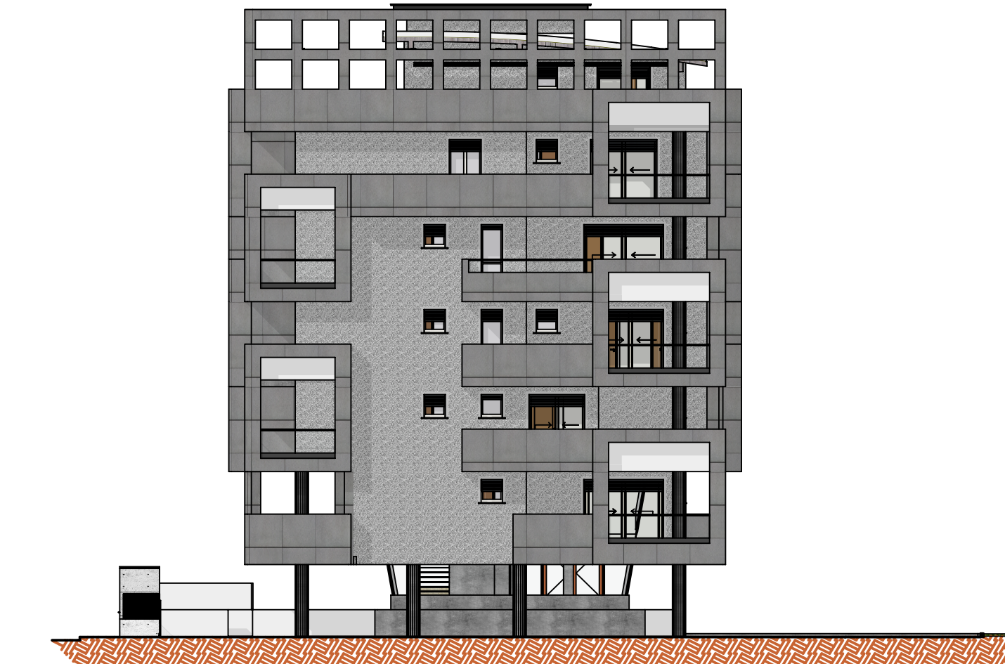
PROSPETTO NORD-OVEST (VISTA DA VIA OBERDAN)
