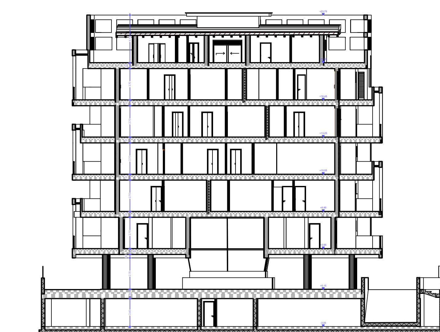
SEZIONE A-A
